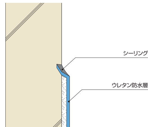
出巾木
