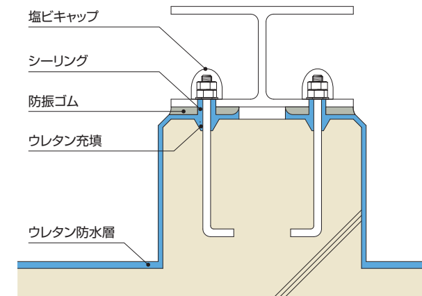
基礎架台
