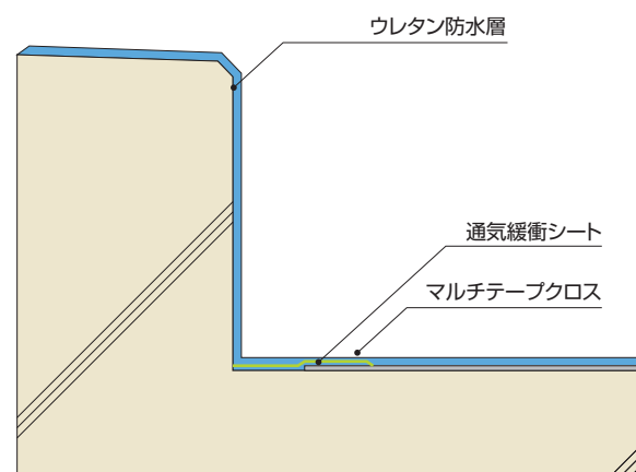
パラペット
