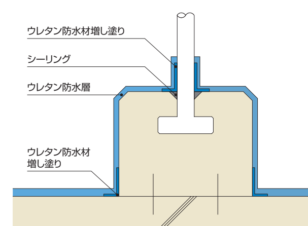
フェンス基礎
