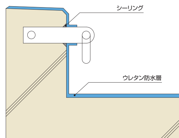
パラペット丸環まわり
