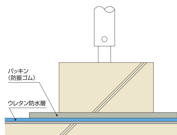
置き基礎
