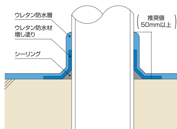
貫通パイプ
