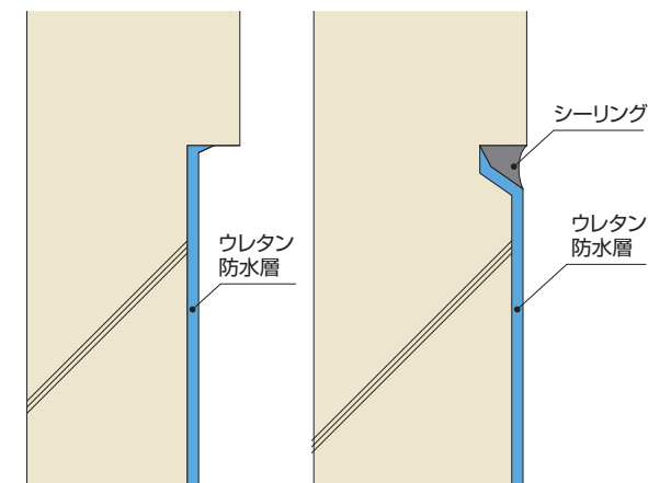
入巾木
