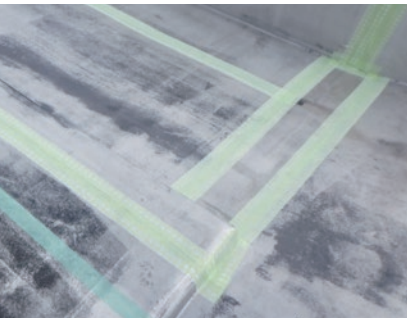
既存シート防水ジョイント部に マルチテープクロス貼付け
